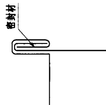
巻締め部詳細図
